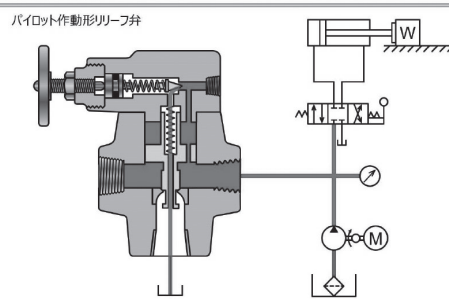
2. リーフ弁
